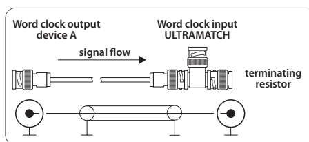
図 5.6: ULTRAMATCH PRO におけるワードクロック入力のアンバランス方式接続方法 (終末端)
