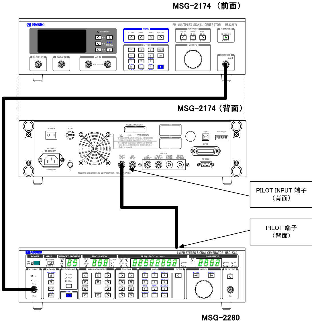
接続図 2
