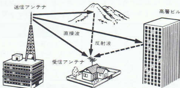
マルチパスの起きる原因
